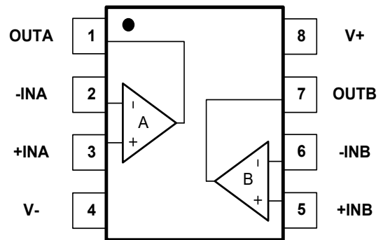
Fig. 5-7. OSU6722: T8 (TSSOP8) Package
