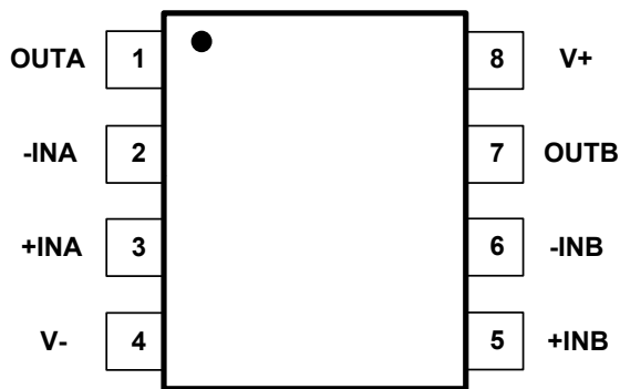
Fig. 5-6. OSU6722: S8 (SOP23-8) Package
