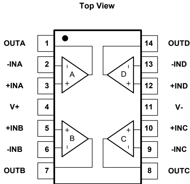
Fig.5-8. OSU6724: TD (TSSOP14) Package
