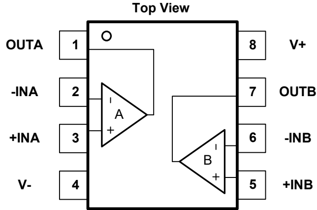
Fig.5-4. OSU6052: P8(SOP8) Package
