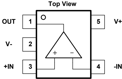
Fig.5-1. OSU6051: C5(SC70-5) Package
