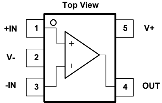
Fig.5-2. OSU6051: BC5(SC70-5) Package
