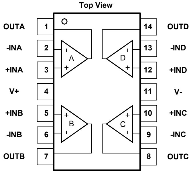
Fig.5-5. OSU6054: TD(TSSOP14) Package
