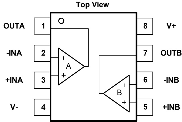
Fig.5-4. OSU6022: P8(SOP8) Package
