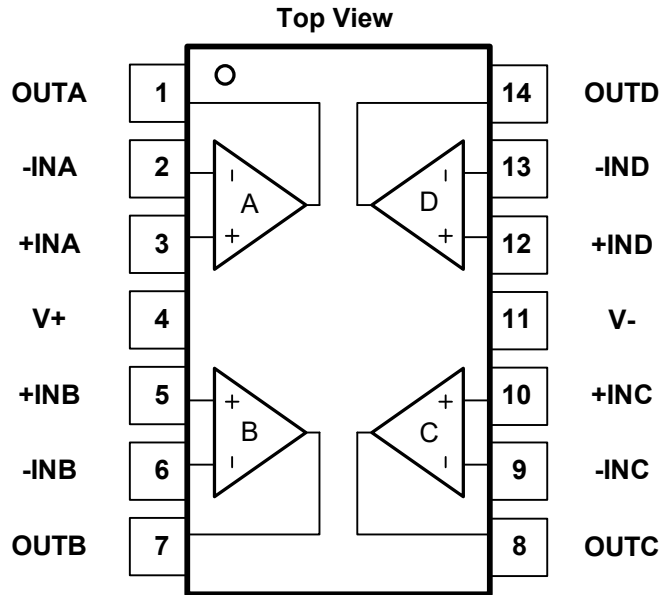
Fig.5-5. OSU6024: TD(TSSOP14) Package
