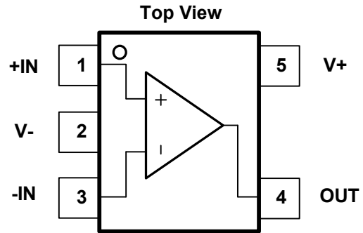
Fig.5-2. OSU6021: BC5(SC70-5) Package OSU6021: BS5(SOT23-5) Package
