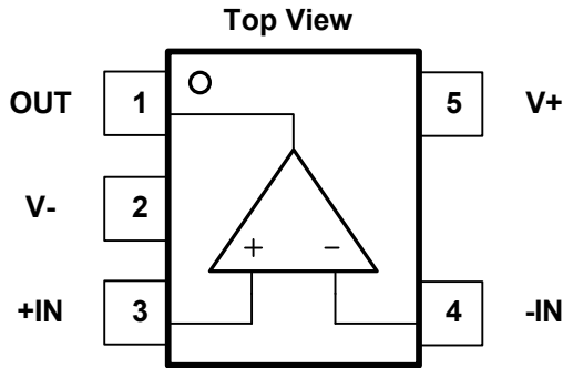
Fig.5-1. OSU6021: C5(SC70-5) Package OSU6021: S5(SOT23-5) Package
