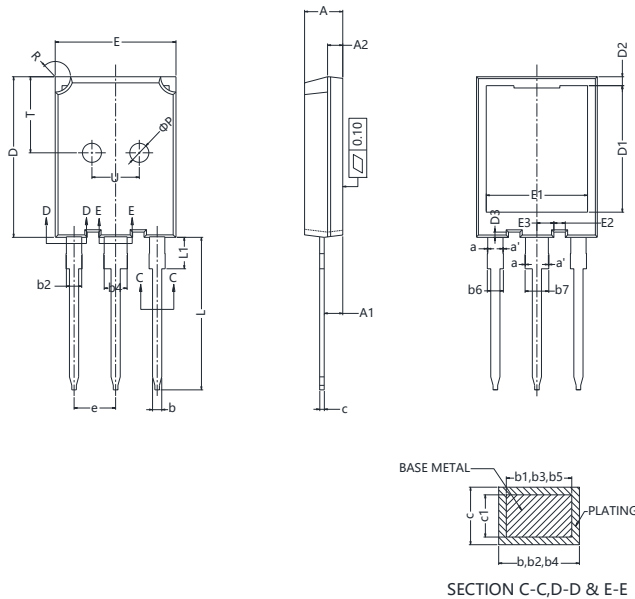
SECTION C-C, D-D &amp; E-E
